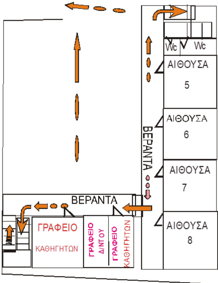
Κάτοψη 1 ου Ορόφου
